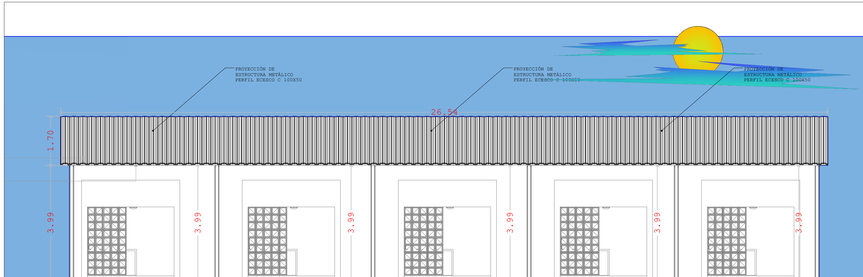
FACHADA OESTE GENERAL ZONA DE COMIDAS ESCALA ----- 1:75
