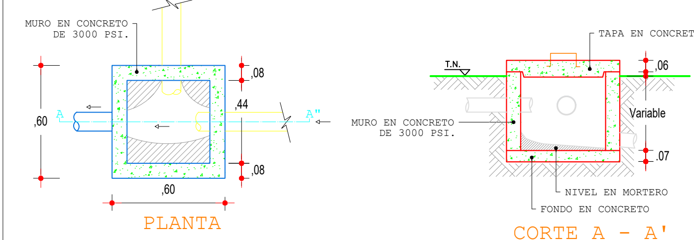
DETALLE DE REGISTRO SANITARIO ESCALA ----- 1:20
