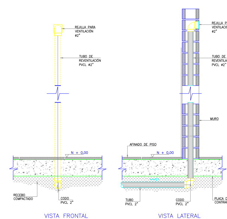
DETALLE INST. SANITARIA REVENTILACION ESCALA ---- 1:20
