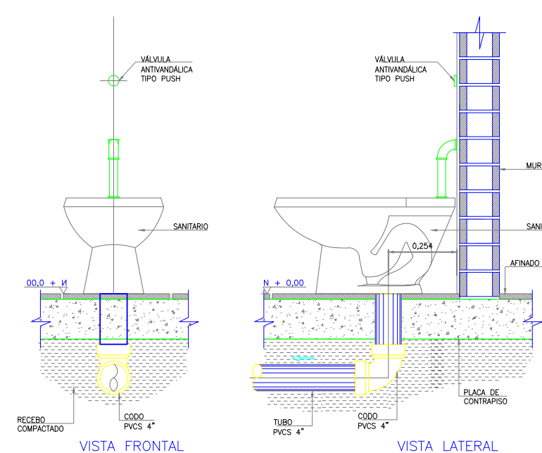
DETALLE INST. SANITARIA SANITARIO ESCALA ---- 1:20
