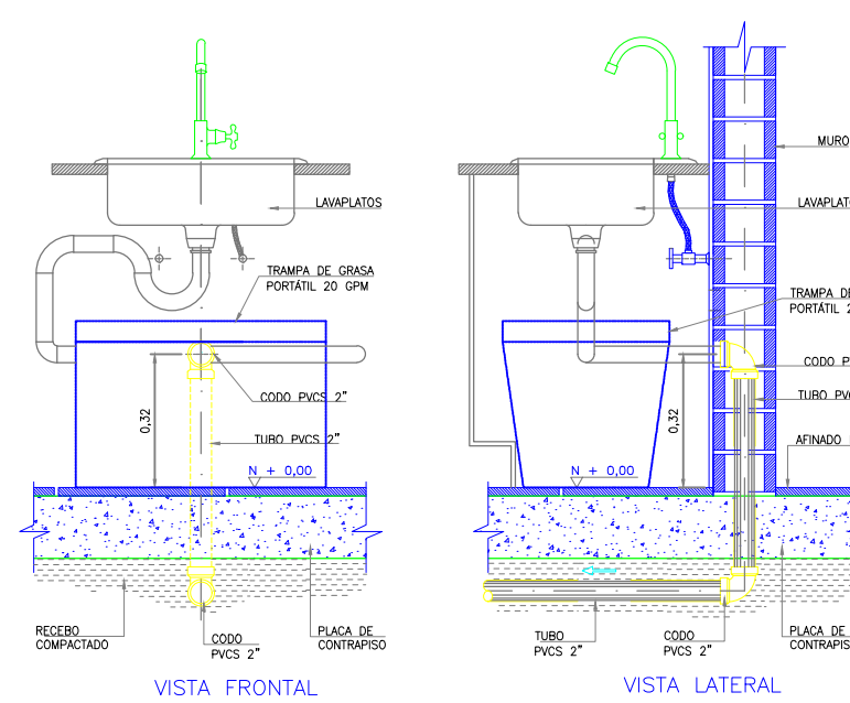
DETALLE INST. SANITARIA LAVAPLATOS ESCALA ---- 1:20
