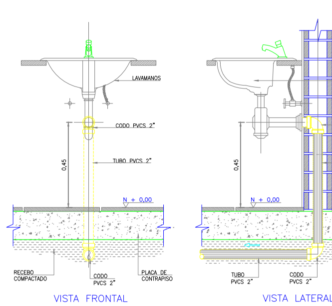
DETALLE INST. SANITARIA LAVAMANOS ESCALA ---- 1:20
