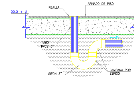
DETALLE INST. SANITARIA SIFÓN DE PISO ESCALA ---- 1:10
